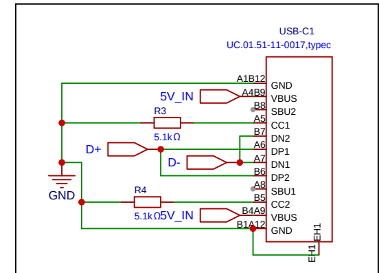
USB-C
