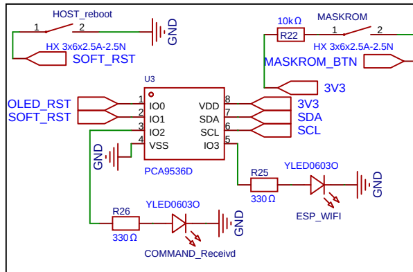
Boutons et Leds d'activité
